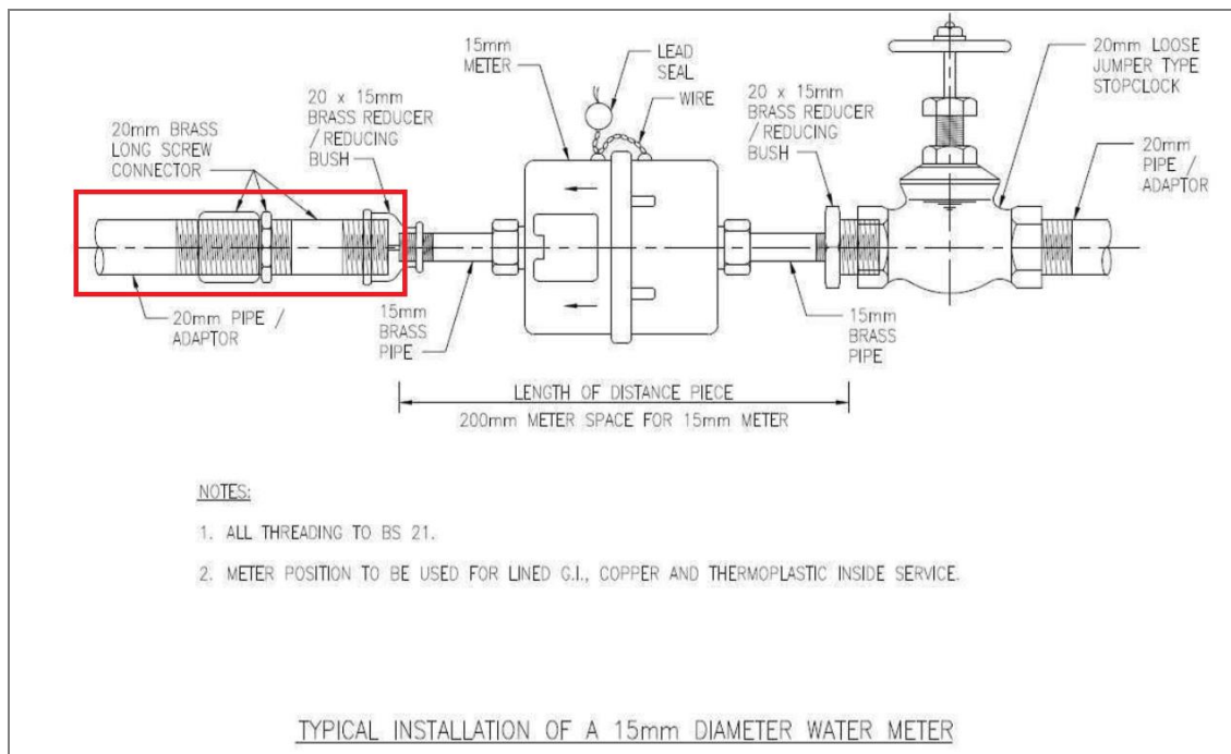
<<樓宇水管工程技術要求>> 圖3 (Fig. 3)
