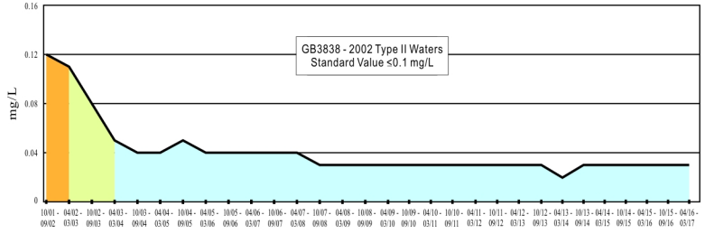
Manganese
