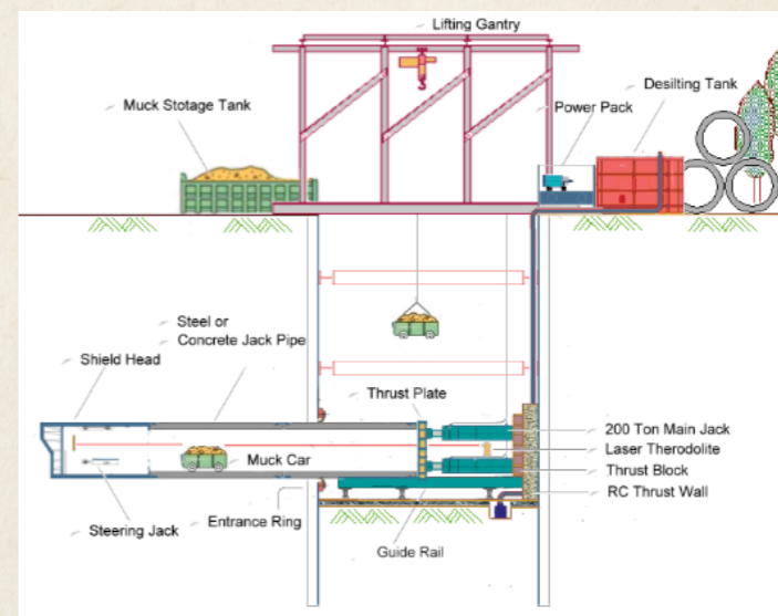
圖三：手挖隧道及豎井（橫切面）
